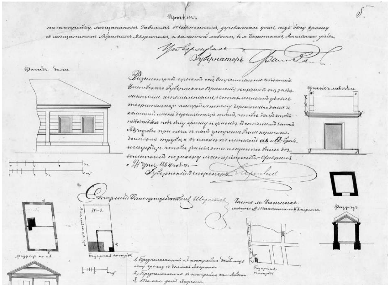
Проект строительства деревянного дома Тиктина Завеля и каменной лавки в м. Чашники, 1884 г. (ГАВО. Ф. 907. Оп. 6. Д. 3. Л. 1)
